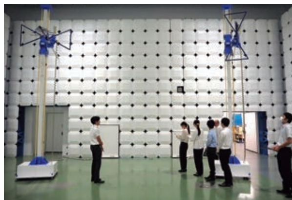
大型電波暗室
